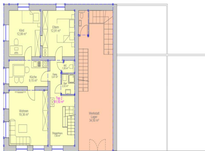
Anlage 8 Grundriss Obergeschoss 1 (Achtung, ohne Maßstab)
